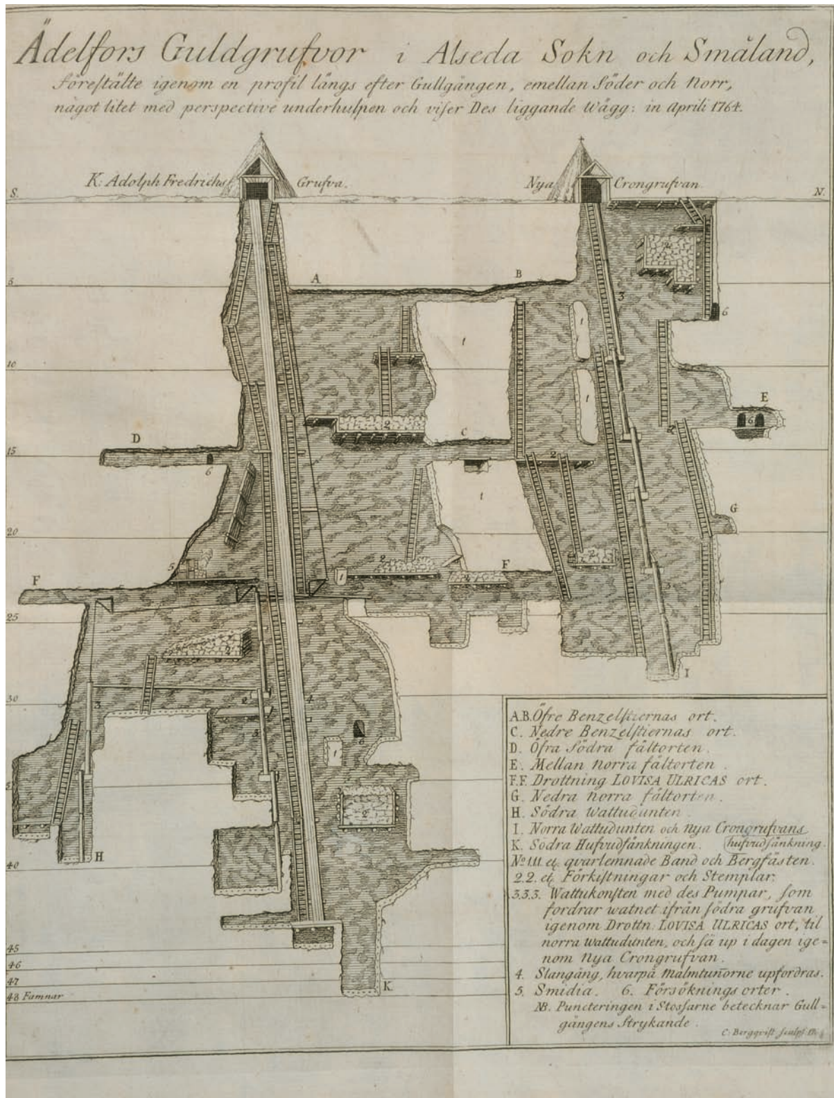
Genomskärning av Ädelfors gruva 1764. Aufriss der Grube Ädelfors 1764.
